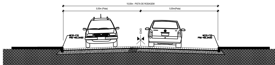
SEÇÃO TIPO DE BLOCO INTERTRAVADO - RUA HELMUTH GUILHERME JUNGBLUT
